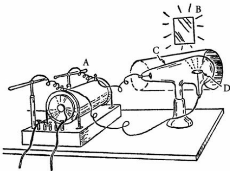
Fig. 21. El aparato de rayos X utilizado por Röntgen consistía en: (A) bobina inductora de alto voltaje; (B)
