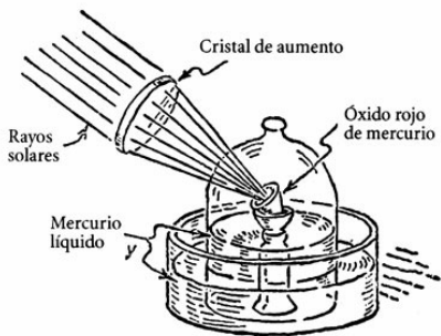
Fig. 7. Los experimentos de Lavoisier fueron ilustrados en sus Elementos de
