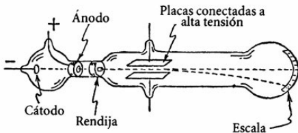
Fig. 20. El tubo de rayos catódicos permitió a Thomson medir la desviación de los haces electrónicos en campos eléctricos de intensidad conocida. El haz pasaba entre las placas, cuyo campo desviaba a los electrones, desplazando sus puntos de choque a lo largo de la escala.
