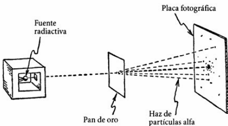
Fig. 23. El experimento de Rutherford condujo al concepto de núcleo, y abrió las puertas a la moderna física nuclear. Las partículas alfa emitidas por la fuente radiactiva se desviaban al pasar a través de un pan de oro. El grado de desviación quedaba registrado cuando las partículas chocaban con la placa fotográfica.
