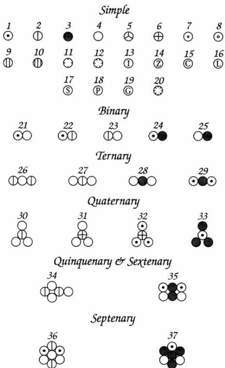
Fig. 9. Símbolos de Dalton para
