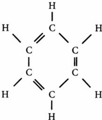
benceno
