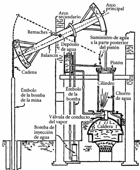
Fig. 5. La máquina de bombeo de Newcomen, que funciona a presión atmosférica. El agua pulverizada en el interior del cilindro condensa el vapor, creado un vacío. El pistón descende en el vado, para volver hasta arriba del émbolo por una nueva inyección de vapor.
