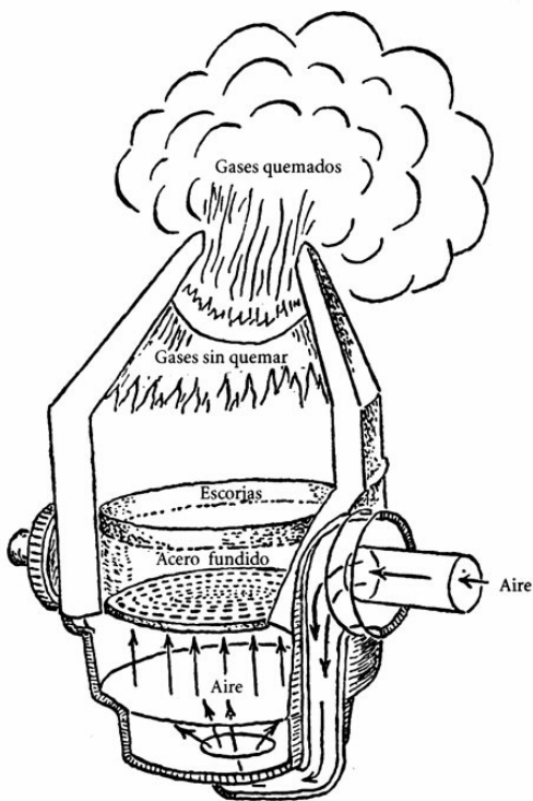
Fig. 19. El convertidor de Bessemer
