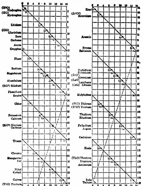
Fig. 14. Un trazo en espiral fue el resultado que obtuvo Béguyer de Chancourtois, en 1862, al ordenar los
