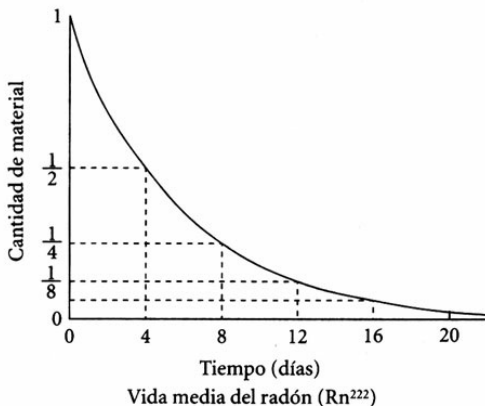
Fig. 22. La vida media del radón se determina midiendo las cantidades de material que quedan al cabo de intervalos de tiempo iguales. La representación es la curva exponencial asintótica, y = e^{-ax} .
