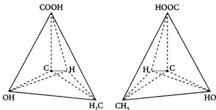
Fig. 11. El enlace tetraédrico de los átomos de carbono permite dos configuraciones de los átomos en los compuestos, siendo una de ellas la imagen especular de la otra. Este modelo muestra las disposiciones en imagen especular de la molécula de ácido láctico, \text{CH}_3\text{CHOCCO}_2\text{H} .
