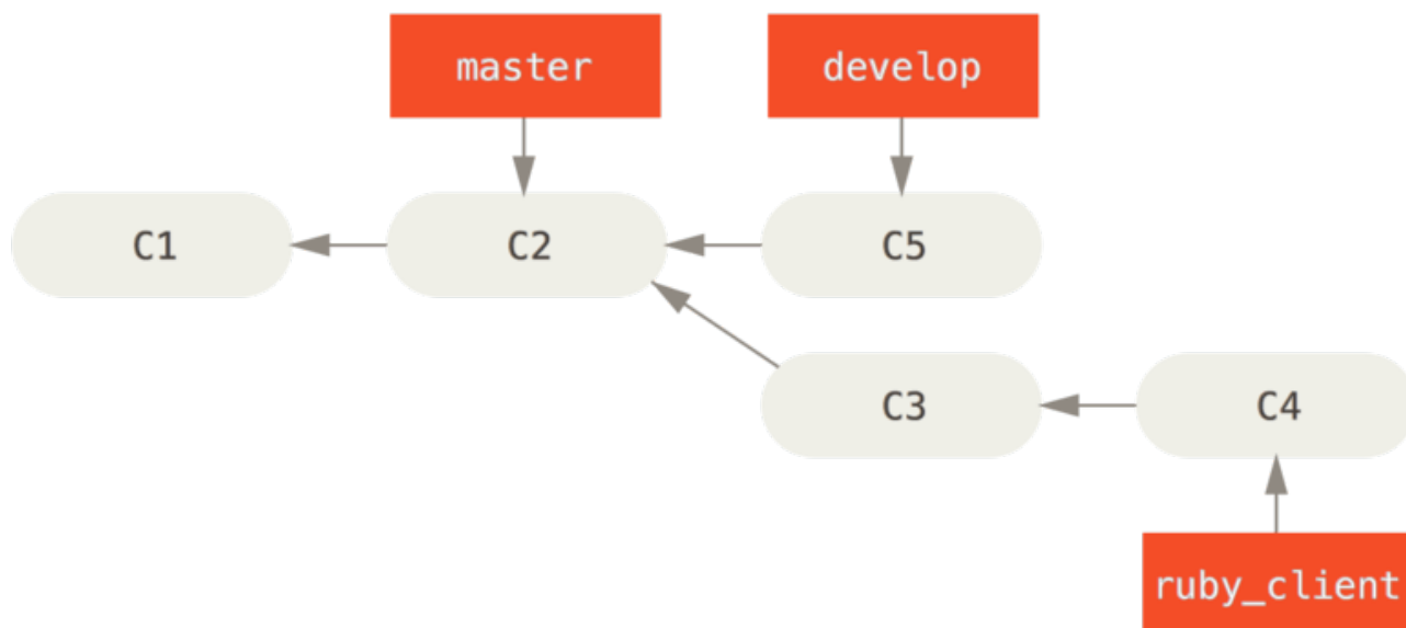
Figure 75. Antes de integrar una rama puntual.
