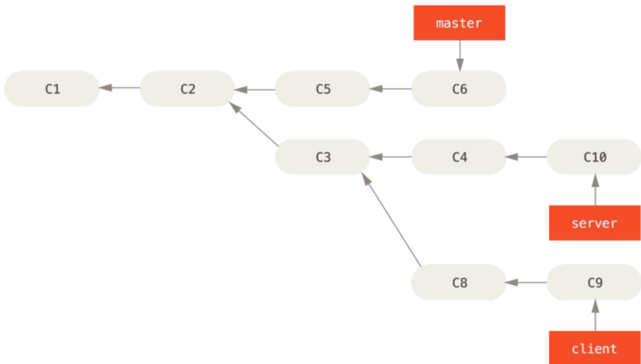
Figure 39. Un historial con una rama puntual sobre otra rama puntual
