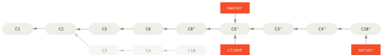
Figure 42. Reorganizando la rama server sobre la rama master
